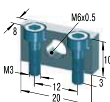
固定支架
