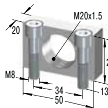
固定支架
