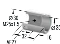
限位套筒
