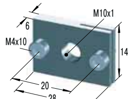
矩形法兰
