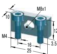
固定支架
