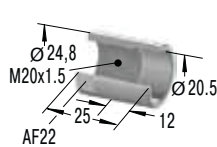
限位套筒
