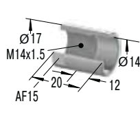
限位套筒
