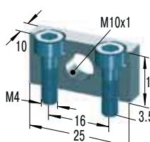
固定支架
